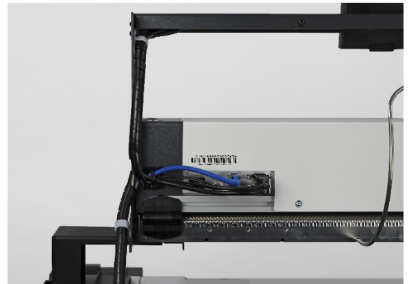
Vista posterior de los conectores y las guías de cable
